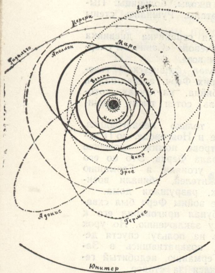
Орбиты некоторых астероидов
